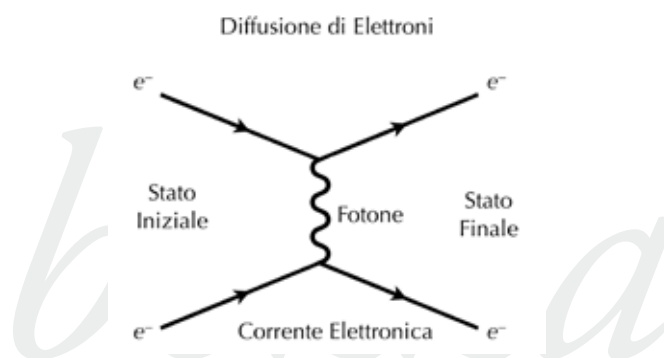
Figura 0.1. Schema di diffusione di elettroni mediato da un fotone, mediatore dell'interazione elettromagnetica
