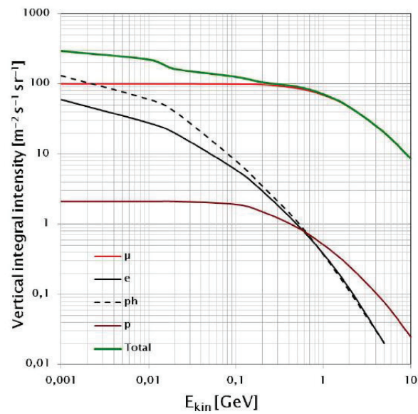
Figura 15.5: Flusso medio dei raggi cosmici a livello del suolo integrato in energia al di sopra di una data soglia, a latitudine 40°.
