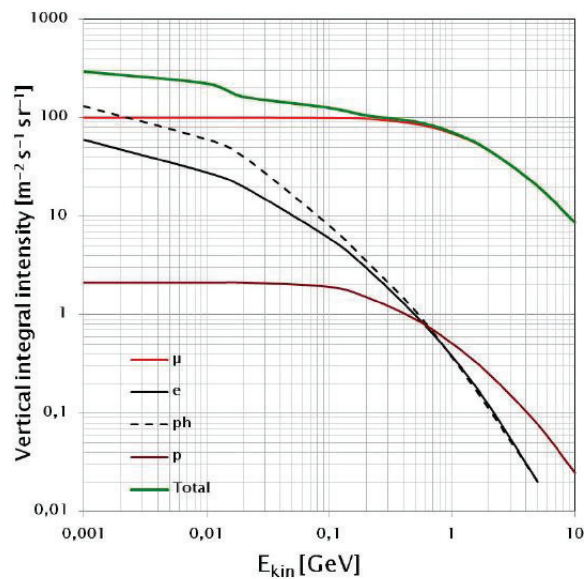
Figura 15.3: Flusso medio dei raggi cosmici a livello del suolo integrato in energia al di sopra di una data soglia, a latitudine 40°.
