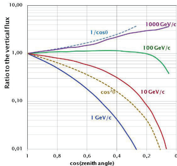
Figura 15.4: Distribuzione angolare dei muoni cosmici a livello del suolo.
