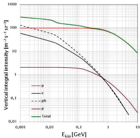
Figura 15.9: Flusso medio dei raggi cosmici a livello del suolo integrato in energia al di sopra di una data soglia, a latitudine 40°.
