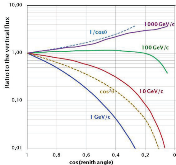
Figura 15.10: Distribuzione angolare dei muoni cosmici a livello del suolo.
